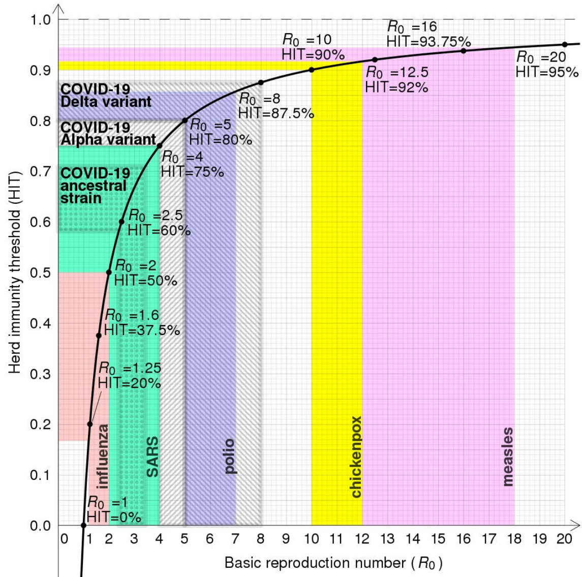
Figura 1. Relación entre el Número básico de reproducción ( R_0 ) y el umbral de inmunidad
